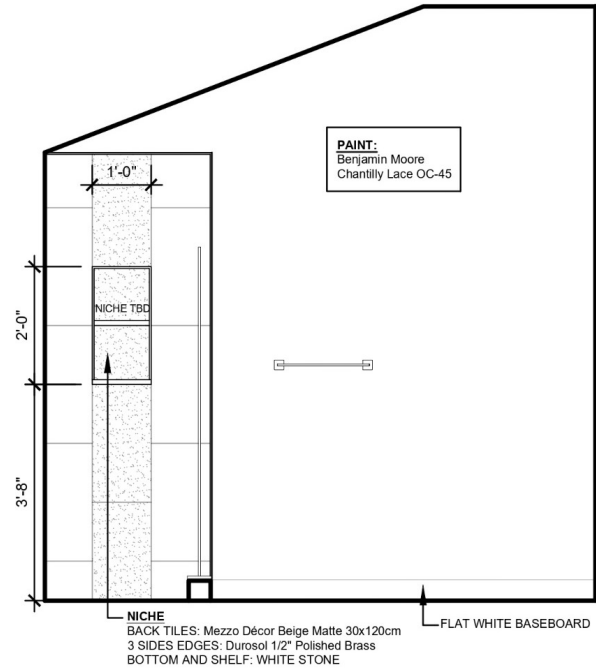
ELEVATION 3
