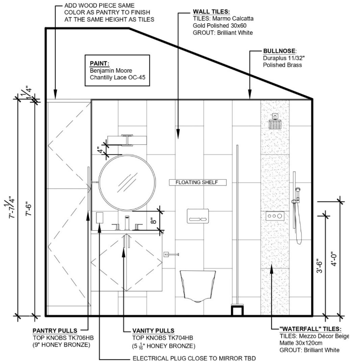
ELEVATION 1
