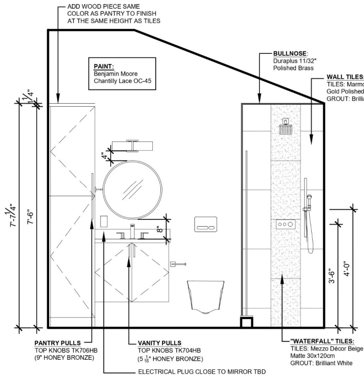
ELEVATION 1
